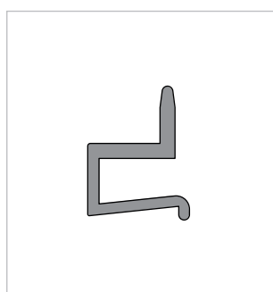
Griffleiste (Standard Unikat)
