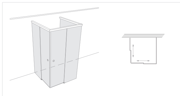
Unikat 133 softslide
